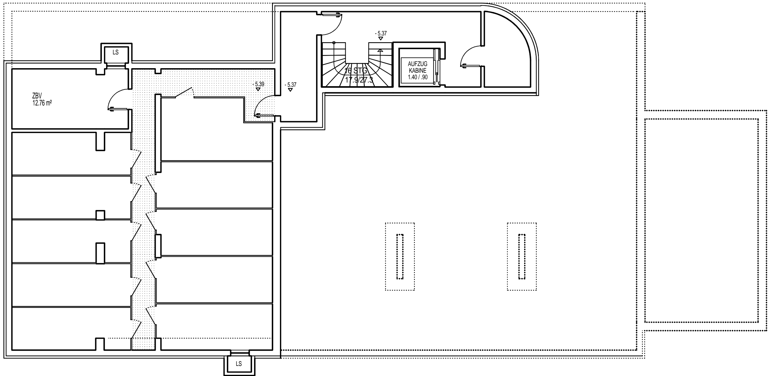
2. UNTERGESCHOSS
